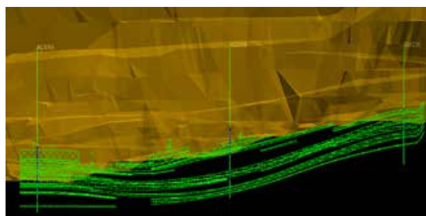
Төв блокийн урд хэсгийн нүүрсний үеийн зүсэлт /2017-12-31 өдрийн байдлаар/
